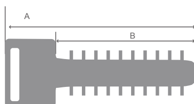
Cheville pour collier de câblage
