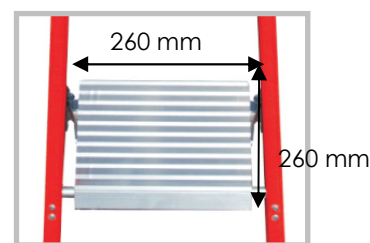
Plateforme supérieure
